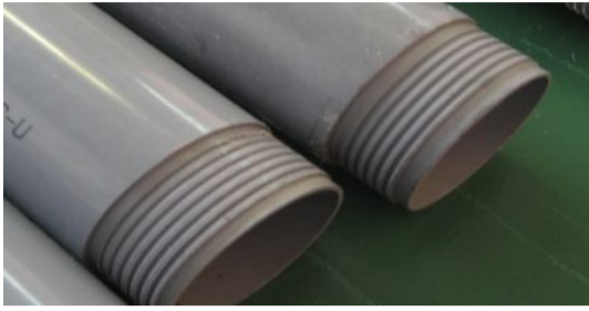
オスネジ形状
