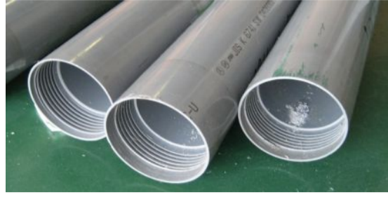
メスネジ形状
