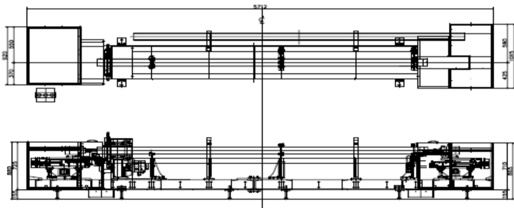
外観形状(5720x1020xH880)
